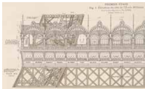
La tour de trois cents mètres, Gustave Eiffel, Société des imprimeries Lemerrier, Paris, 1900. Planches, détail du premier étage © Gallica.BnF.
